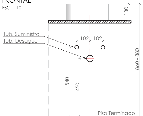
INSTALACIÓN LATERAL ESC. 1:10
